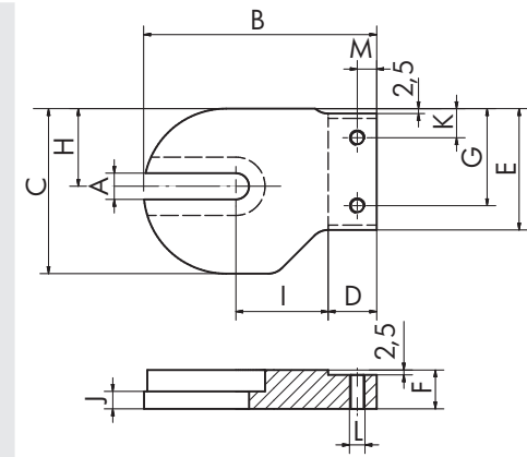
图：右侧支架（A）铝或 VA
