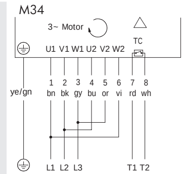
图：3 相，7+2 芯电缆，双电压绕组，三角形接法
