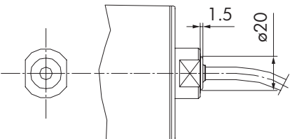
图：直管接头，PU 轴盖
