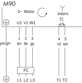
图：3 相，4+2 芯电缆，单电压绕组，星形接法
