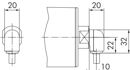
图：弯管接头，高分子聚合物
