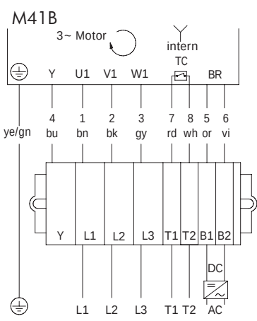
图：带制动，3 相，单电压绕组，星形接法
