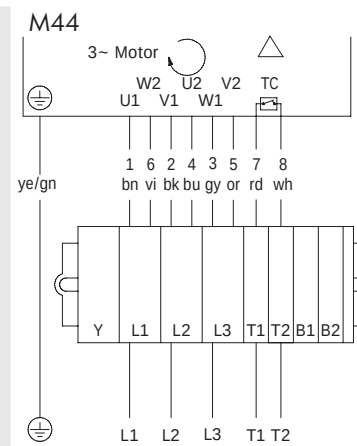
图：3 相，双电压绕组，三角形接法
