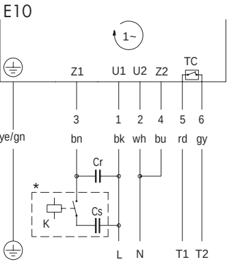
图：单相，7 芯电缆
