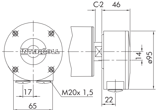
图：接线盒，铝
