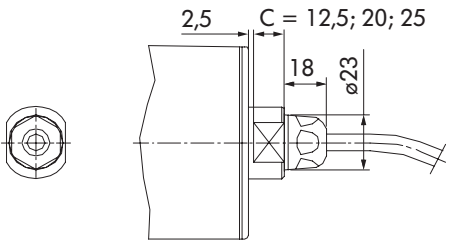
图：直插接头连接，符合 IP69k 卫生清洁标准，不锈钢
