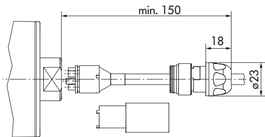
图：用安装工具安装的尺寸
