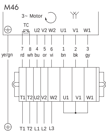
图：3 相，7+2 芯电缆，双速，双星形接法
