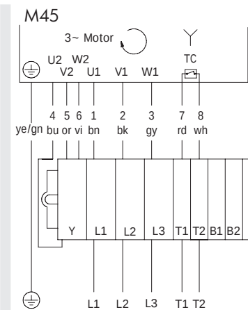
图：3 相，双电压绕组，星形接法
