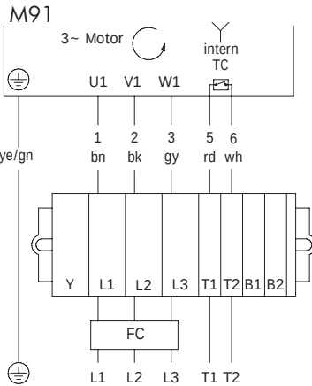
图：3 相，4+2 芯电缆，单电压绕组，星形接法
