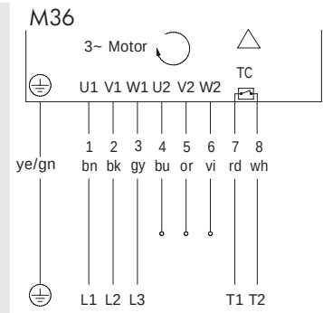
图：3 相，7+2 芯电缆，双速，三角形接法
