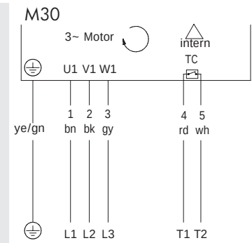
图：3 相，4+2 芯电缆，单电压绕组，三角形接法
