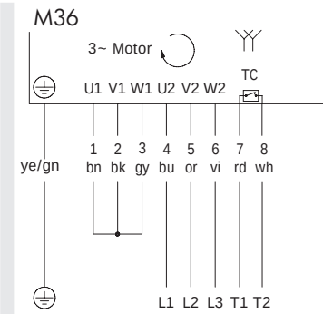
图：3 相，7+2 芯电缆，双速，双星形接法
