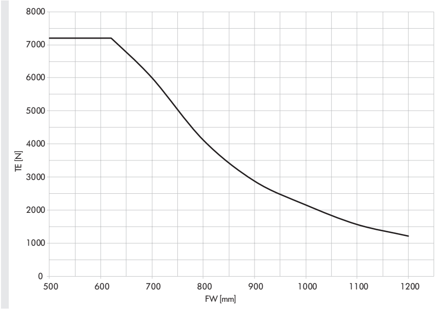
皮带张力图
