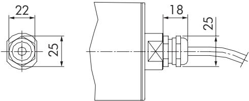
图：直型 EMC 接头，黄铜或不锈钢
